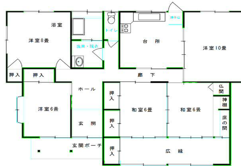
間取図
